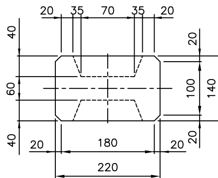
VISTA B-B
