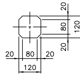
VISTA A-A
